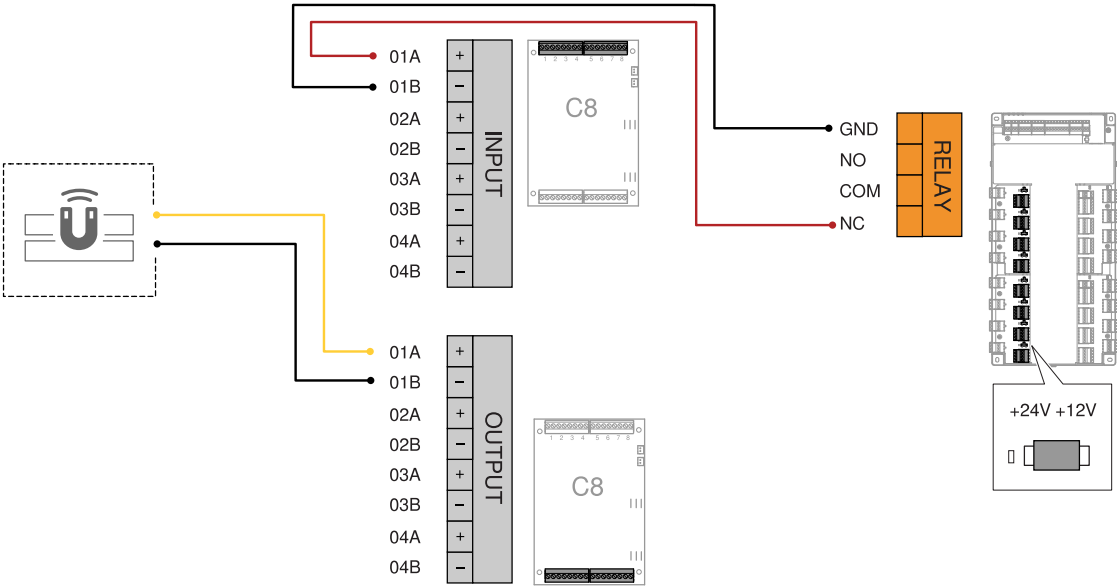
Przełącznik drzwiowy do płyty C8, opcja 2
