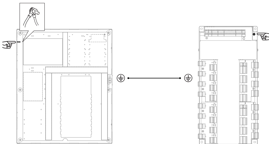
Kontroler drzwiowy do uziemienia obudowy
